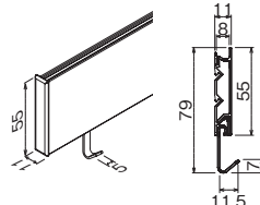
左右にスライドするフック 石こう壁用ピンで取り付け
